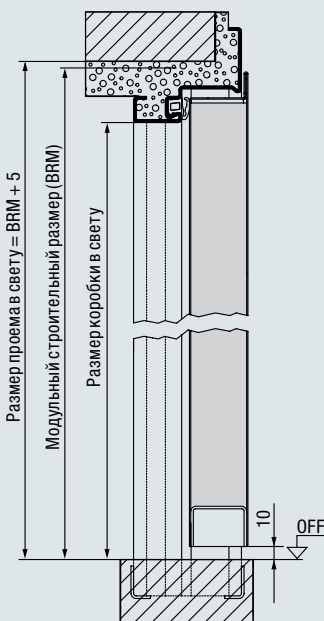
Вертикальный разрез
