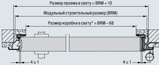
Горизонтальный разрез
